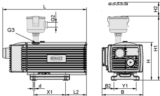
Dati di costruzione EVE-TR-X 25 AC3 VBV
