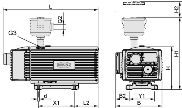
Datos de diseño EVE-TR 25 AC3
