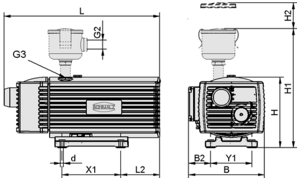
Données de construction EVE-TR 16 AC
