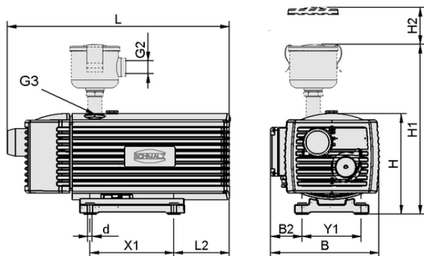
Dati di costruzione EVE-TR 16 AC
