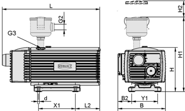
Tasarım verileri EVE-TR 10 AC3
