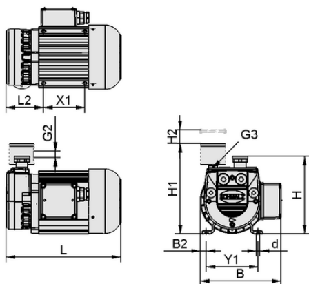
Dati di costruzione EVE-TR 8 AC
