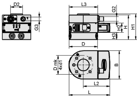
Datos de diseño RECBi 24V-DC NO UNI 1C M12-8
