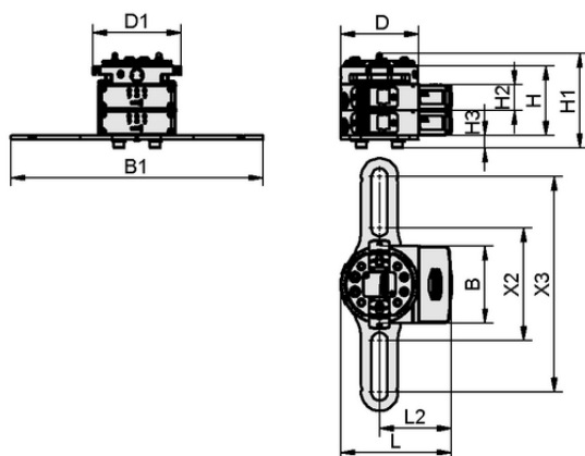
Dati di costruzione RECBi 24V-DC NC PXR-I 2C MATCH
