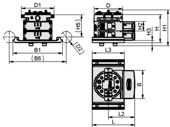
Datos de diseño RECBi 24V-DC NO PXT-2 2C MATCH
