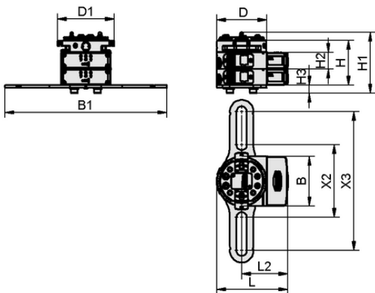
Données de construction RECBi 24V-DC NO PXR-I 2C MATCH
