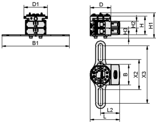
Données de construction RECBi 24V-DC NC PXR-I 1C MATCH
