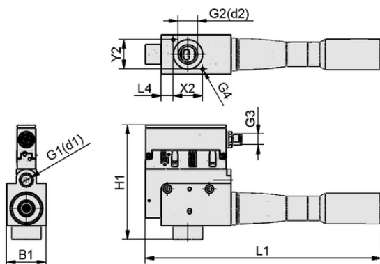
Dati di costruzione SCPSc-L HV 3-20 NO M12-5 PNP
