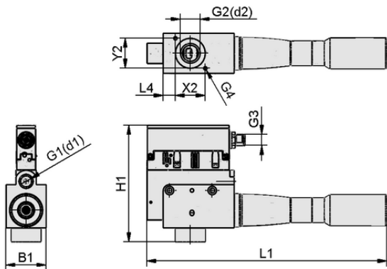
Données de construction SCPSc-L HV 3-20 NO M12-5 PNP
