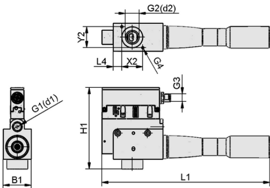
Données de construction SCPSc-L HV 3-20 NC M12-5 PNP
