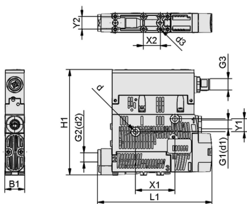
Dati di costruzione SCPSc 2-09 G02 NO M12-5 PNP
