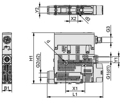
Données de construction SCPSc 2-09 G02 NO M12-5 PNP
