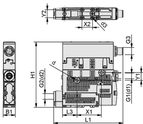
Dati di costruzione SCPSc 07 G02 NC M12-5 PNP
