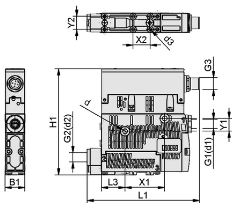
Données de construction SCPSc 07 G02 NC M12-5 PNP
