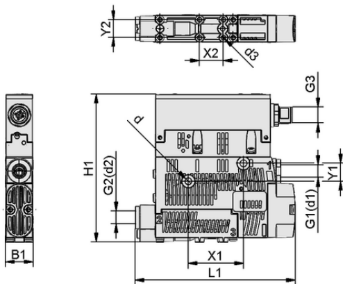
Données de construction SCPSc 2-14 G02 NO M12-5 PNP
