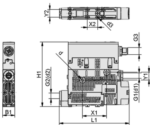
Données de construction SCPSc 2-14 G02 NC M12-5 PNP
