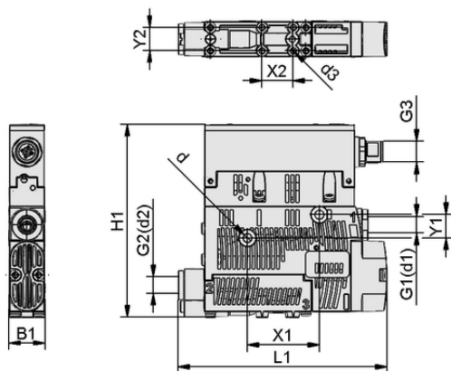
Dati di costruzione SCPSc BY 2-14 G02 NC M12-5 NPN
