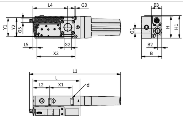
Design data SCPLc 100 HV G SA NO PNP E2D
