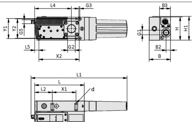
Design data SCPLc 100 HV G SA NC PNP E2C
