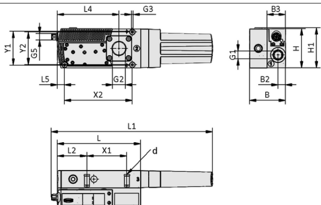
Dati di costruzione SCPLb 100 HV G SA NO PNP E17
