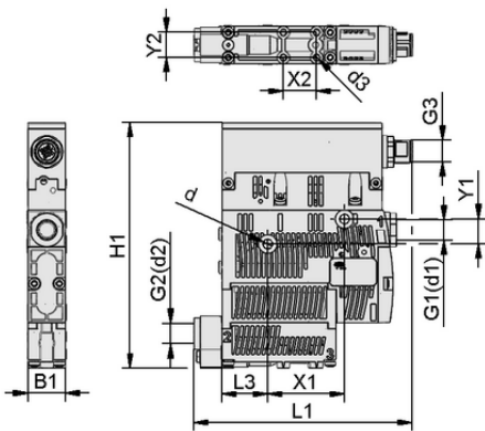
Données de construction SCPSi 15 M G02 IMP M12-5
