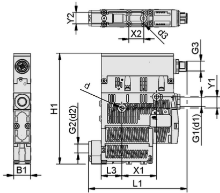
Tasarım verileri SCPS 07 M G02 NC M12-5 NPN
