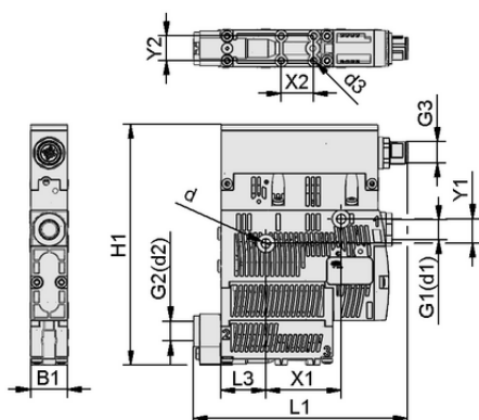
Dati di costruzione SCPS 15 M G02 NC M12-5 PNP
