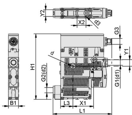
Dati di costruzione SCPS 10 M G02 NC M12-5 PNP
