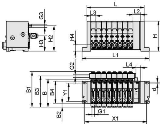
デザインデータ SCTSi PNT 8
