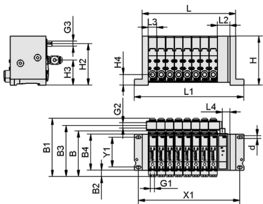
Données de construction SCTSi IOL 8
