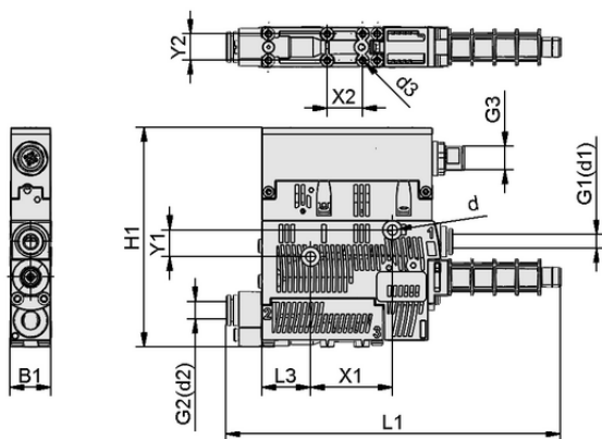
Dati di costruzione SCPS-UHV-HD 11 G02 NO NPN
