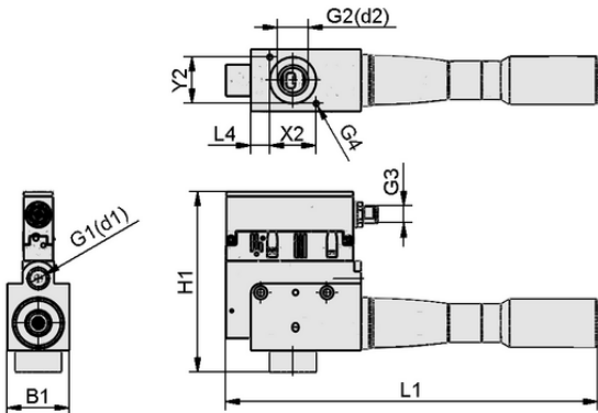
Datos de diseño SCPS-L HV 3-16 NO M12-5 PNP
