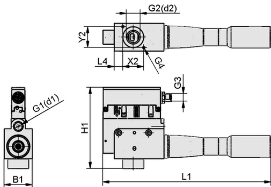
Données de construction SCPS-L HV 3-20 NC M12-5 PNP
