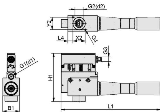
Données de construction SCPSi-L HV 3-16 NC M12-5
