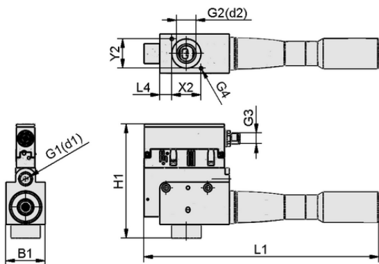
Datos de diseño SCPSi-L HV 3-20 NO M12-5
