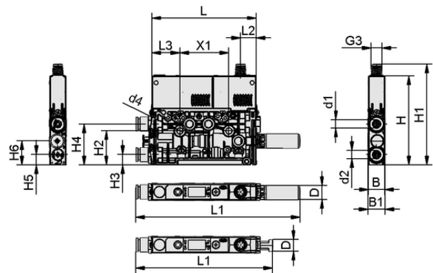
Données de construction SCPMi 03 S01 NC M8-6 ABH
