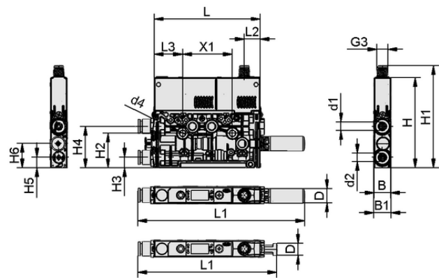
Données de construction SCPMc 05 S01 NO M8-6 NPN AA4
