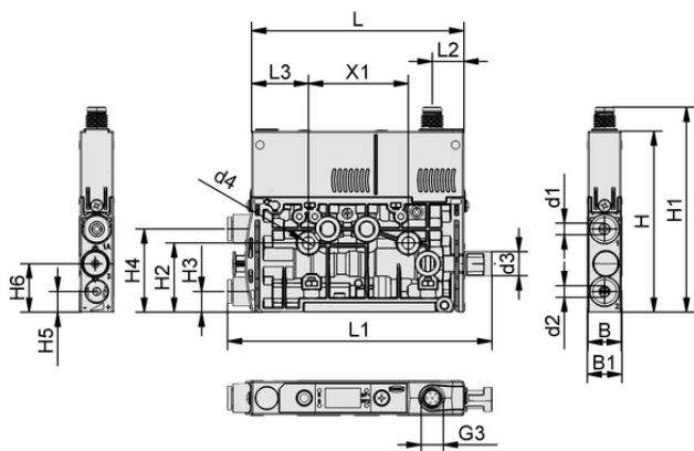
Dati di costruzione SCPMc 03 S01 NO M8-6 NPN AA2
