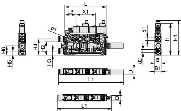
Données de construction SCPMb 05 S01 NC AAD
