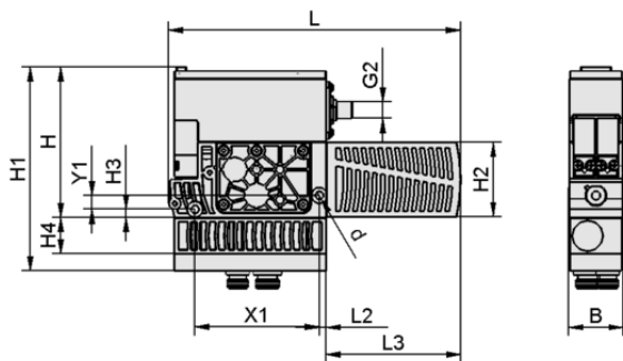
Données de construction SXMPi 30 IMP Q M12-5
