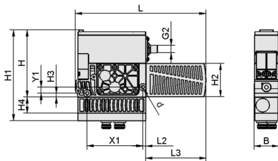
Dati di costruzione SXMPi 25 IMP Q PC M12-5
