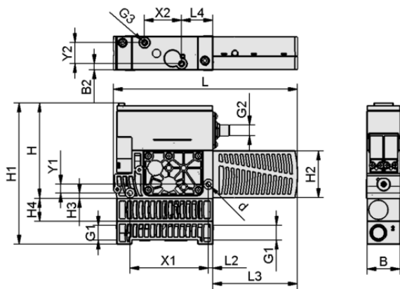
Données de construction SXMPi 25 IMP H PC M12-5
