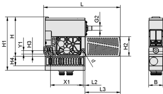
Données de construction SXMPi 30 NC Q PC M12-5
