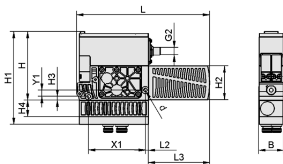
Dati di costruzione SXMPi 25 NC Q M12-5
