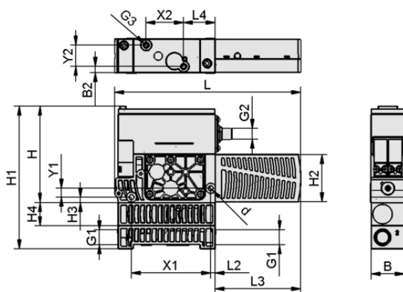
Dati di costruzione SXMPi 25 NC H M12-5
