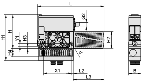
Données de construction SXMPi 25 NO Q M12-5
