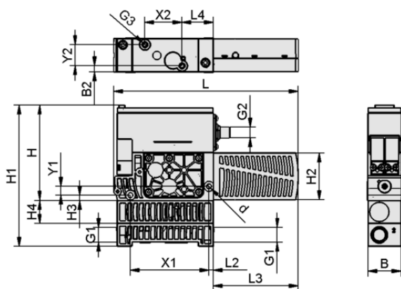
Dati di costruzione SXMPi 25 NO H M12-5
