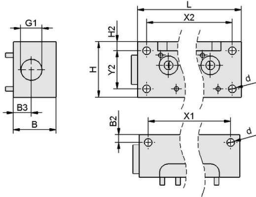
Tasarım verileri GP 8 SCPS 07..15 G2
