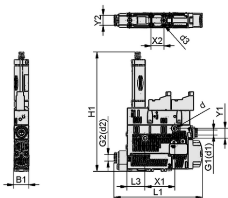
Dati di costruzione SCPSb 2-09 S04 NC VD
