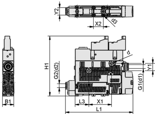
Données de construction SCPSb 2-14 S02 NC
